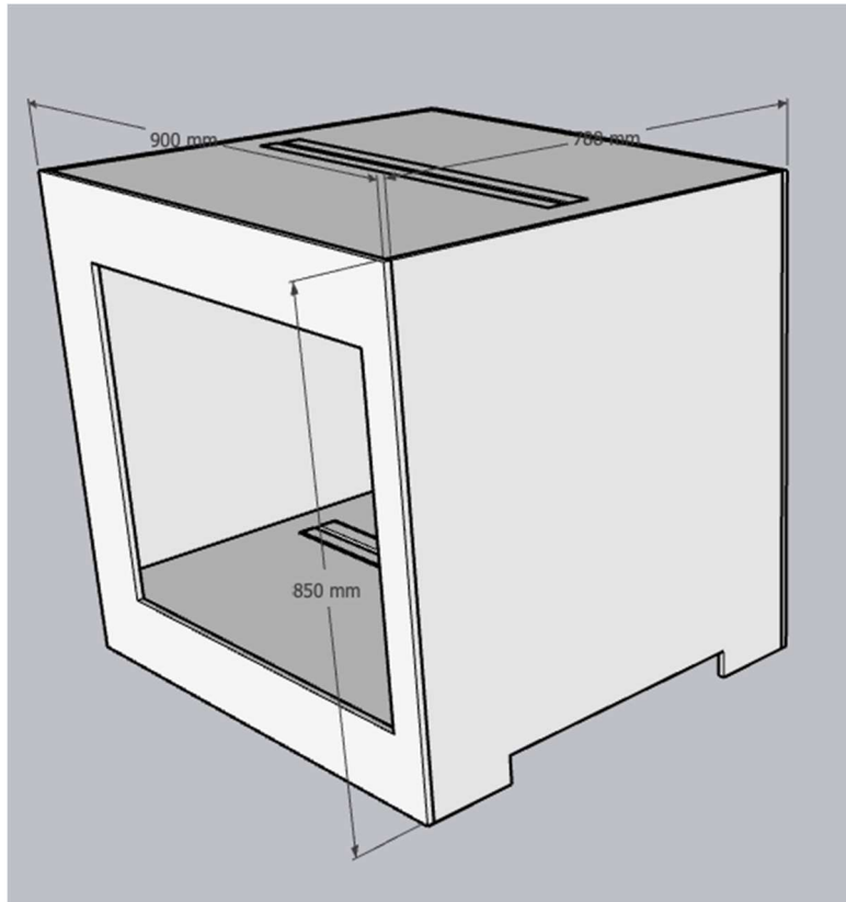
Ryc. 2A. Widok ogólny modułu pod instrumenty automatyczne.
