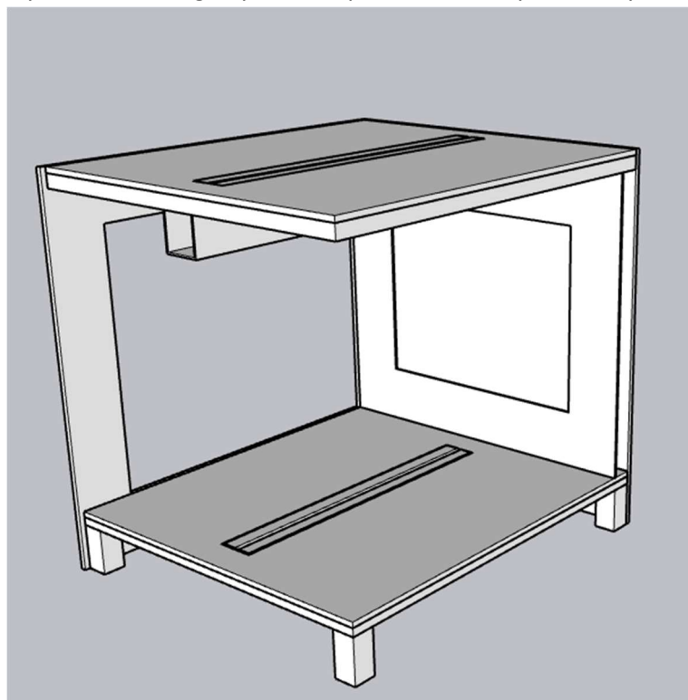
Ryc. 2B. Widok ogólny modułu pod instrumenty automatyczne bez przedniej i bocznej ściany.
