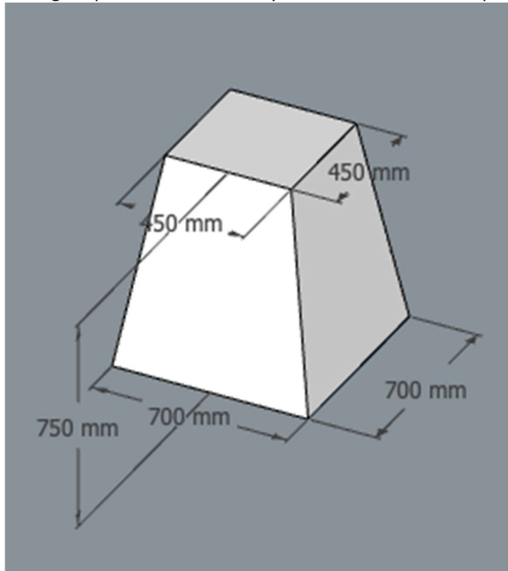
Ryc. 4. Moduł pod robota.
